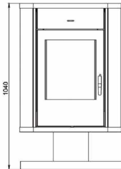
Вид спереди
